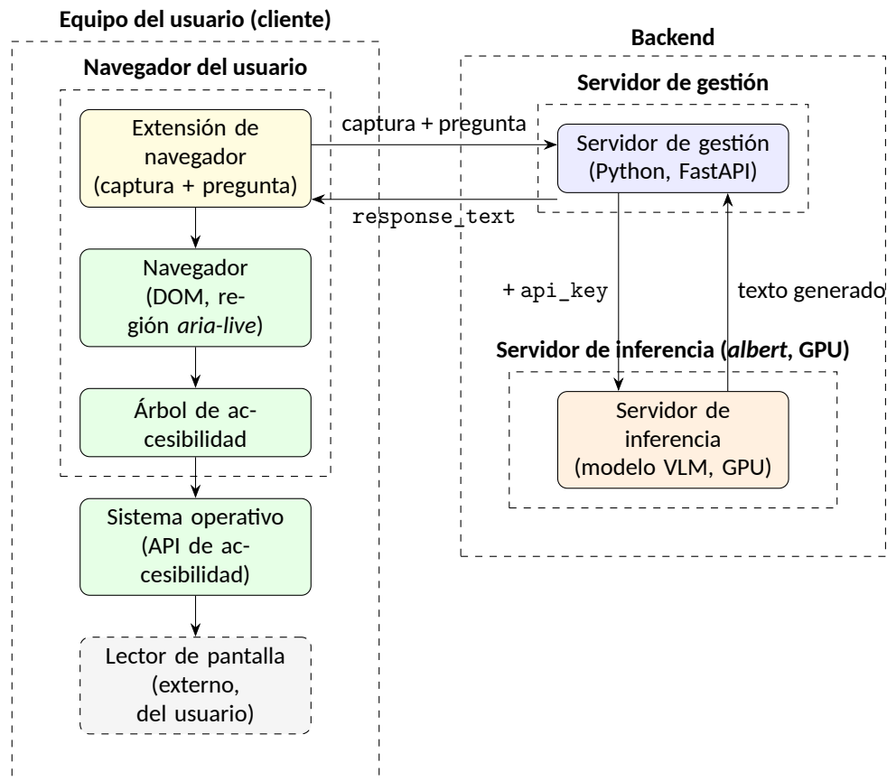
Figura 4: Arquitectura general del relator de pantalla.
